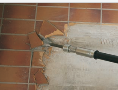
Lösen von Fliesen und Platten
