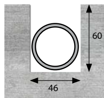
Schlitzten von Rohrkanälen
